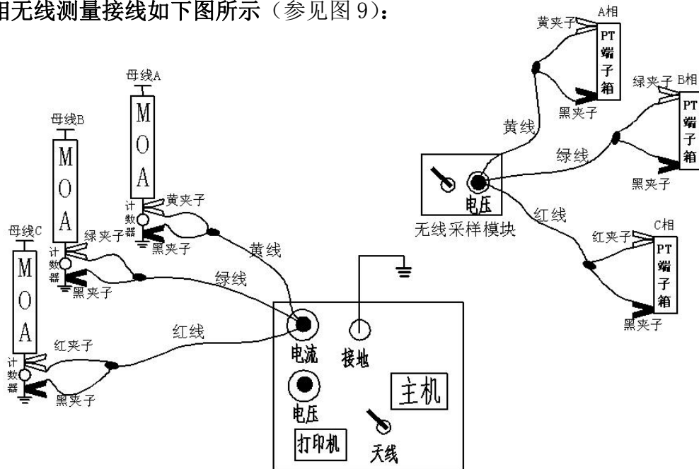
图 9 三相测量无线传输接线示意图
