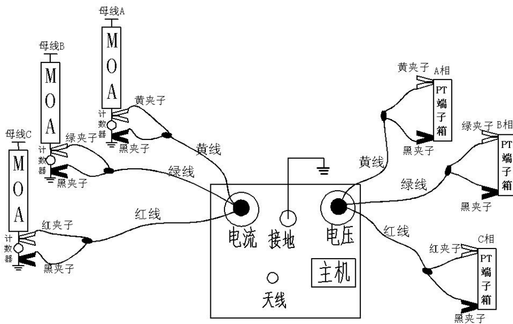
图 8、三相测量有线传输接线示意图
