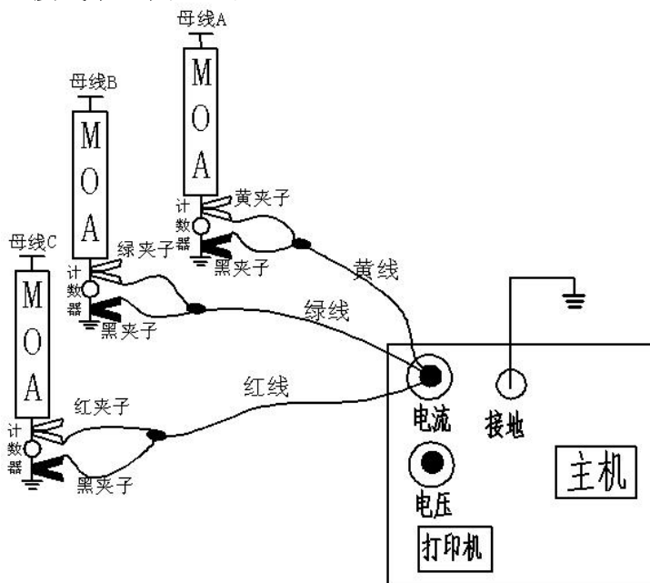
图 10 无 PT 接线示意图
