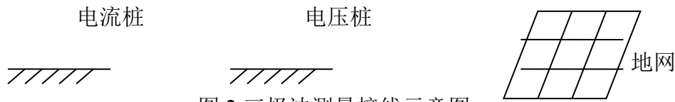
图 2 三极法测量接线示意图
