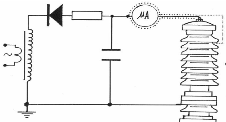
图 7b 排除试品 C_X 表面影响接线图
